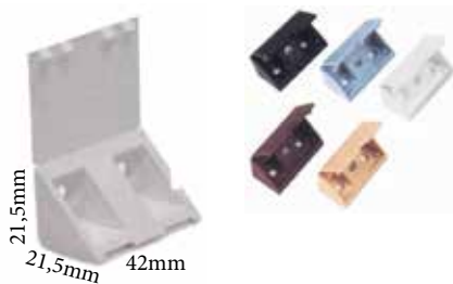
ΓΩΝΙΑ ΠΛΑΣΤΙΚΗ ΣΥΝΔΕΣΗΣ PLASTIC CORNERS
